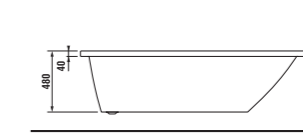
Instalační rozměry vany bez panelu
